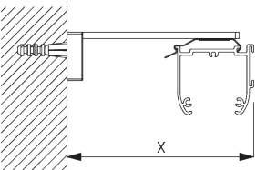
Square Smart Fix SG 11210 - SG 11215 et support SG 2616: Vis SG 10395 (M4x6) nécessaire.
