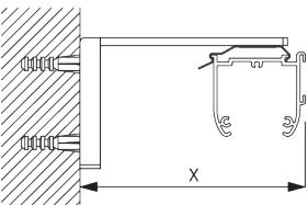
Smart Fix SG 11200 - SG 11205 et support SG 2616: Vis SG 10395 (M4x6) nécessaire.
