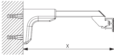
Universal Smart Fix SG 11154 - SG 11156 et support SG 3603: Vis SG 10277 (M4x12) nécessaire.
