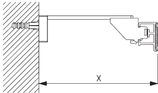
Square Smart Fix SG 11210 - SG 11215 et support SG 3603: Vis SG 10492 (M4x8) nécessaire.
