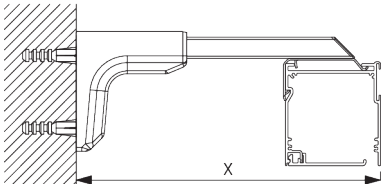
Universal Smart Fix SG 11154 - SG 11156 et support SG 2521: Vis SG 10492 (M4x8) nécessaire.
