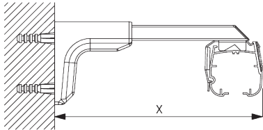
Universal Smart Fix SG 11154 - SG 11156 et support SG 2302: Vis SG 10492 (M4x8) nécessaire.
