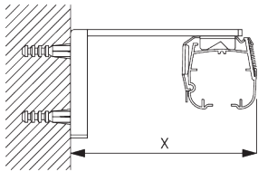
Smart Fix SG 11200 - SG 11205 et support SG 2302: Vis SG 10395 (M4x6) nécessaire.
