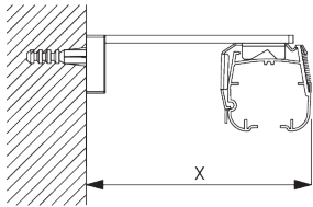
Square Smart Fix SG 11210 - SG 11215 et support SG 2302: Vis SG 10395 (M4x6) nécessaire.
