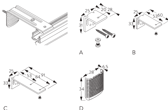
A: Supports-équerre 28 mm (M1) vis incluses
