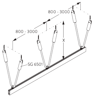
SG 6501: Les suspensions V procurent une stabilité latérale complémentaire.
