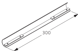
SG 6521 Pièce de raccord
